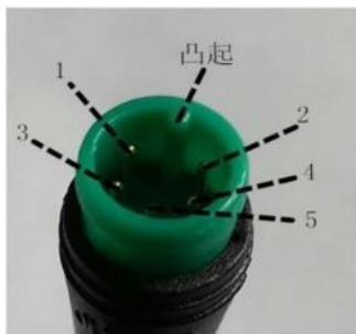
仪表出线端
